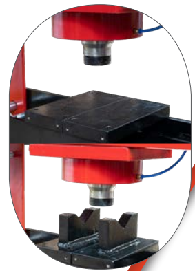
Variable Auflagefläche
