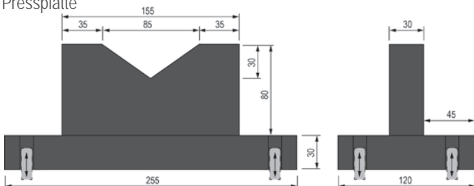
Pressplatte
