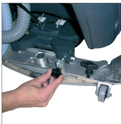
2. Einstellen der Absaugleiste, so dass die Maschine keine Wasserstreifen zieht.
