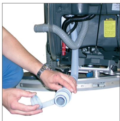
1. Entleeren des Frisch- und Abwassertanks.
